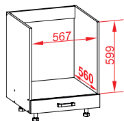
DP-60/82-K rozměry korpusu: š. 600 mm v. 820 mm hl. 560 mm
