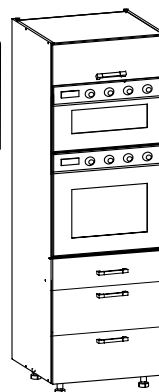
DPS-60/207-2SMB(STB)/SMB(STB)/O rozměry korpusu: š. 600 mm v. 2066 mm hl. 560 mm
