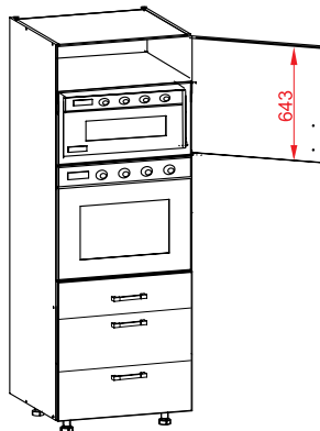
DPS-60/207-2SMB(STB)/SMB(STB)/P(-L) rozměry korpusu: š. 600 mm v. 2066 mm hl. 560 mm
