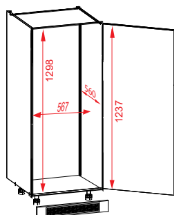
DL-60/143 rozměry korpusu: š. 600 mm v. 1430 mm hl. 560 mm
