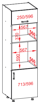
DPS-60/207-P/O rozměry korpusu: š. 600 mm v. 2066 mm hl. 560 mm
