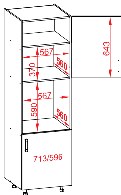
DPS-60/207-P/P rozměry korpusu: š. 600 mm v. 2066 mm hl. 560 mm
